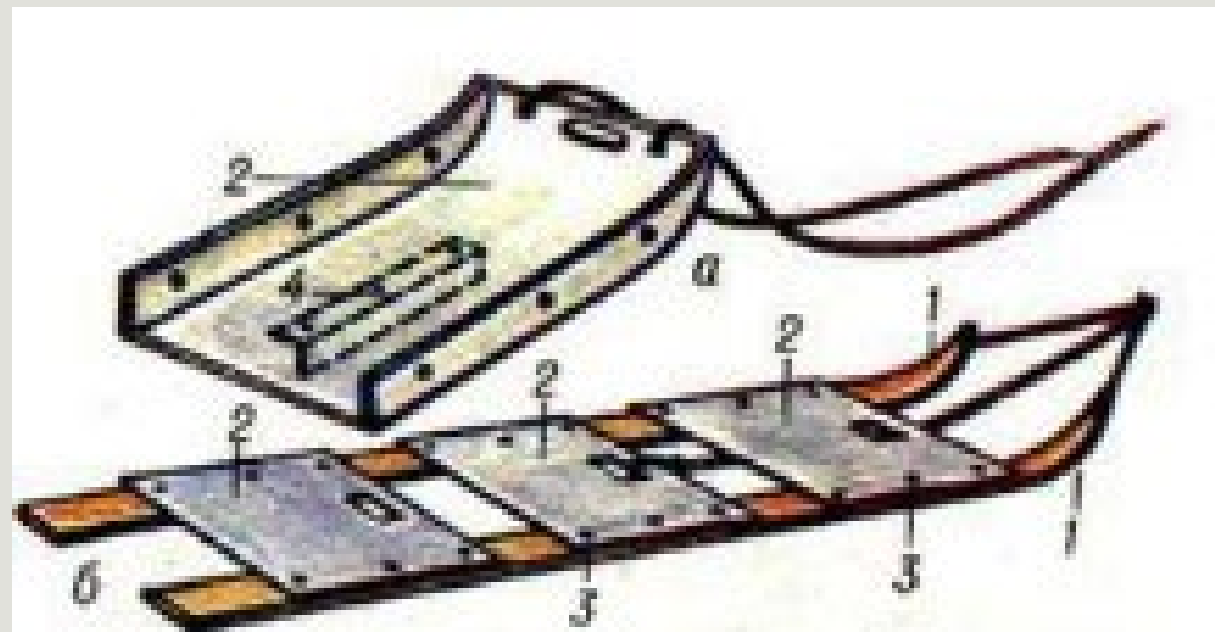
Рис. 3. Волокуша из листов дюралюминия: а — из одного листа; б — из нескольких листов; 1 — лыжи; 2 — дюралевый лист; 3 — крепёжные шурупы.
